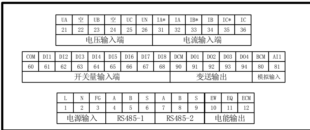
图5 96×96多功能电力仪表端子布置图2
