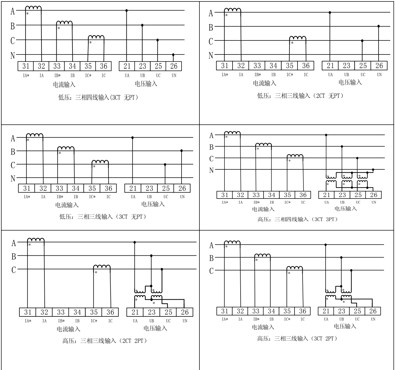
图 7 典型输入信号接线图
