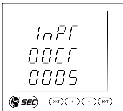
图8 编程示例
