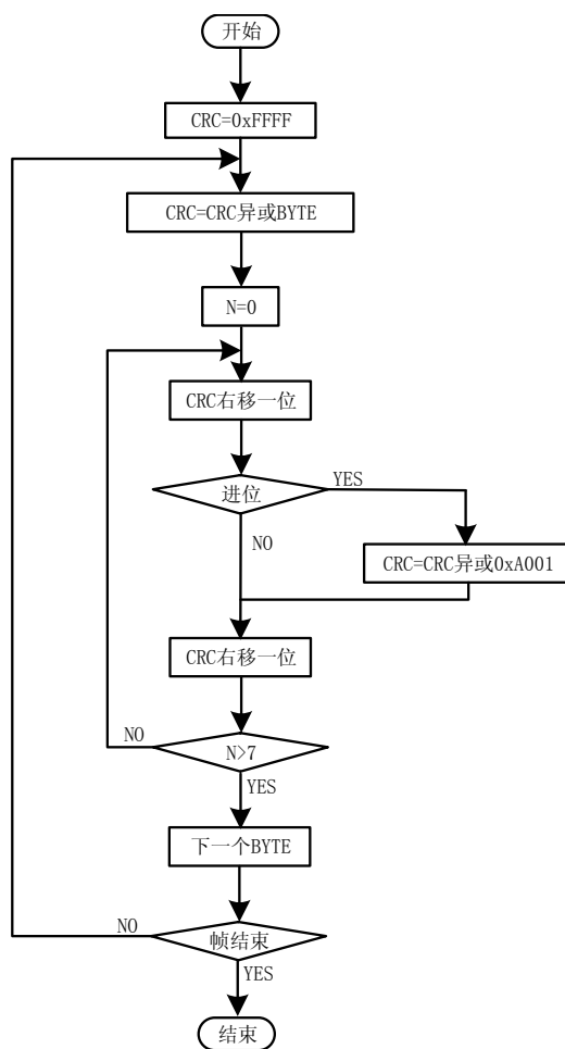
图15 CRC16校验
