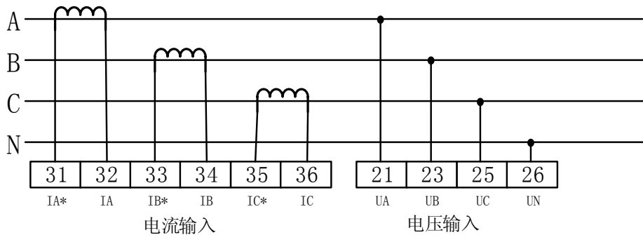
图5 96×96多功能电力仪表端子布置图2
