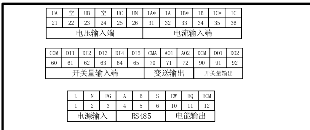
图6 72×72多功能电力仪表端子布置图2
