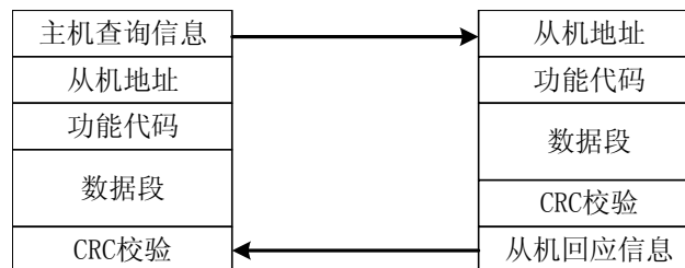
图14 主机与从机之间的通讯
