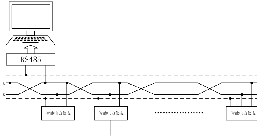
图13 T型网络连接方式
