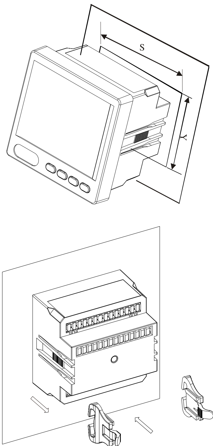
图 2 安装示意图
