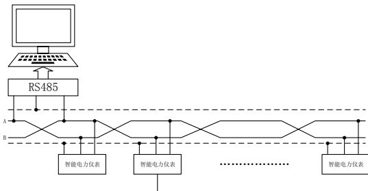
图13 T型网络连接方式
