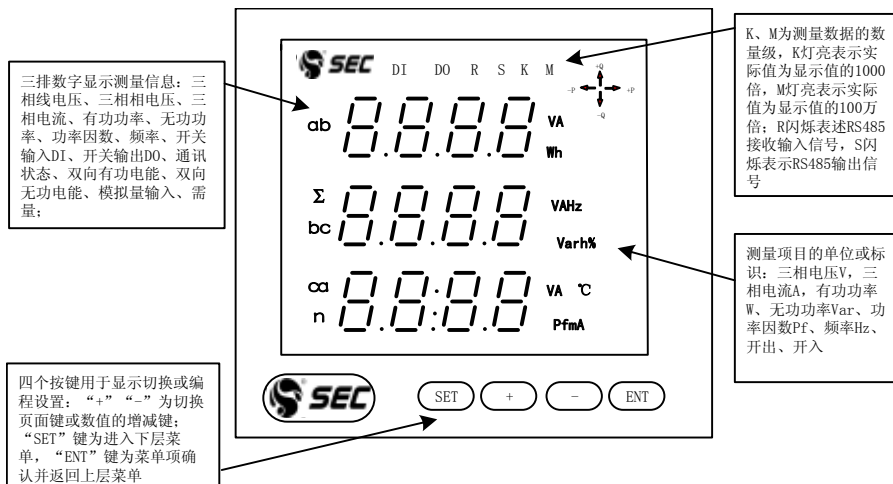
图12 面板说明与测量信息显示
