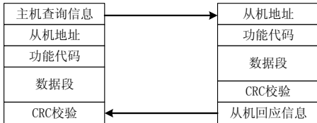
图14 主机与从机之间的通讯
