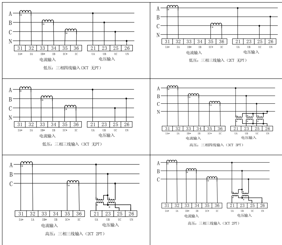
图 7 典型输入信号接线图
