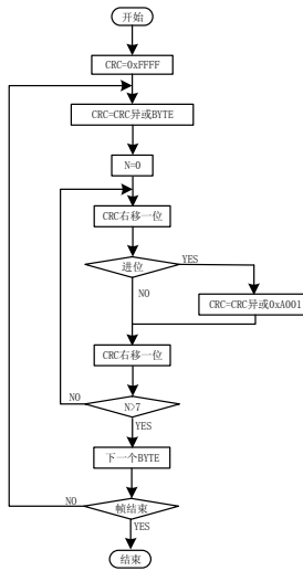
图15 CRC16校验
