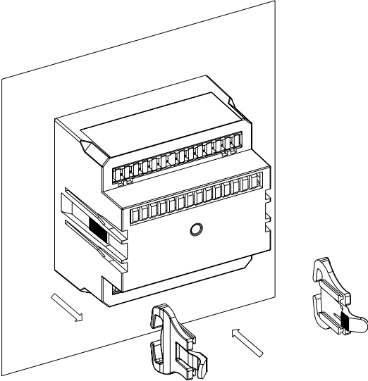
图 2 安装示意图
