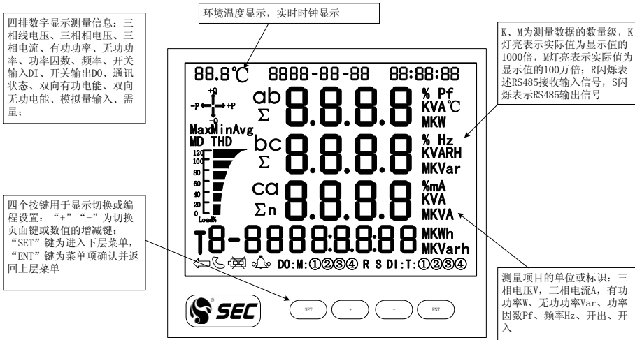
图11 液晶显示内容
