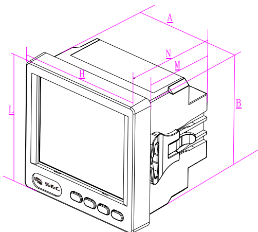
图 1 仪表尺寸
