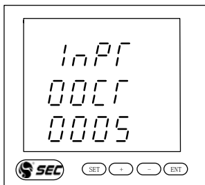
图8 编程示例
